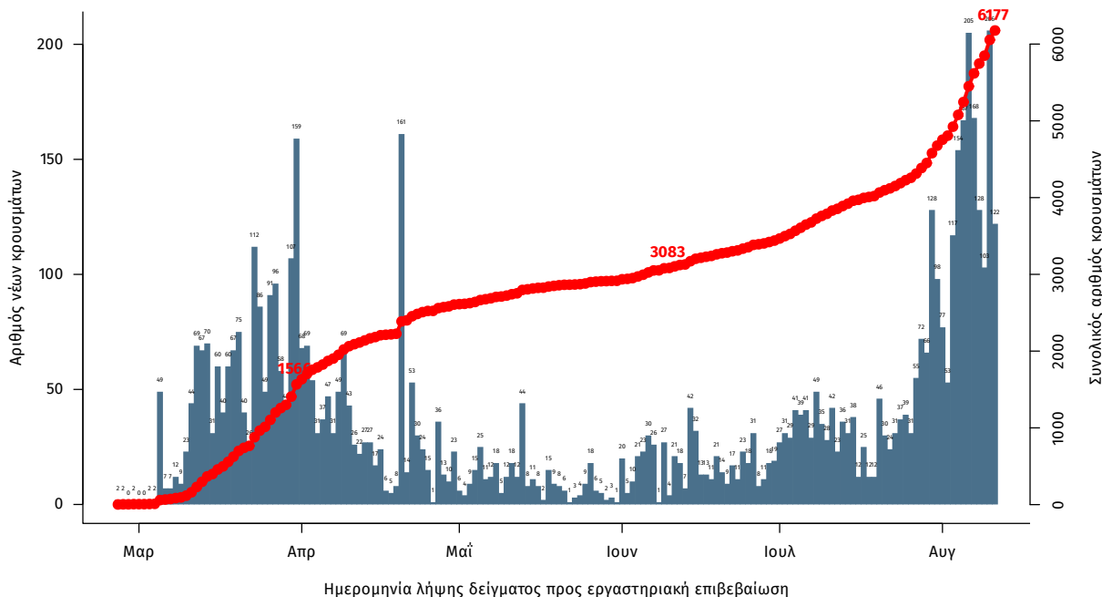
Διάγραμμα 1: Αριθμός εργαστηριακά επιβεβαιωμένων κρουσμάτων COVID-19 στην Ελλάδα, 12 Αυγούστου 2020
