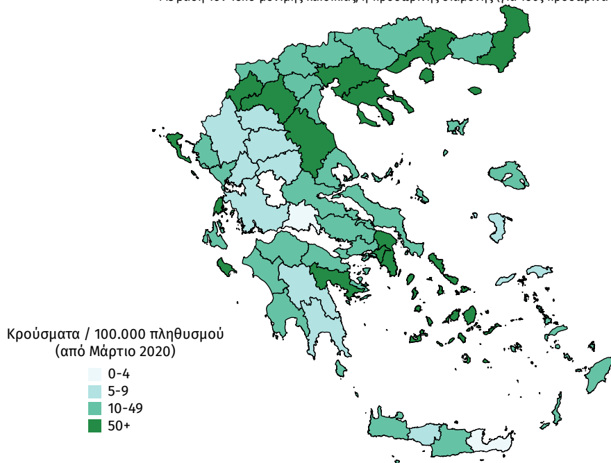
Διάγραμμα 3: Χάρτης αθροιστικής επίπτωσης επιβεβαιωμένων κρουσμάτων COVID-19, 12 Αυγούστου 2020
