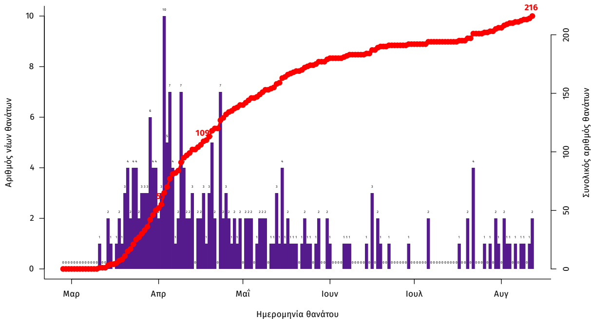
Διάγραμμα 2: Αριθμός εργαστηριακά επιβεβαιωμένων θανάτων με COVID-19 στην Ελλάδα, 12 Αυγούστου 2020
