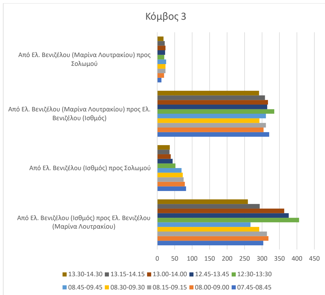
Διάγραμμα 9: Οπτικοποίηση αποτελεσμάτων κυκλοφοριακών ροών (ΜΕΑ/h) στον κόμβο 3
