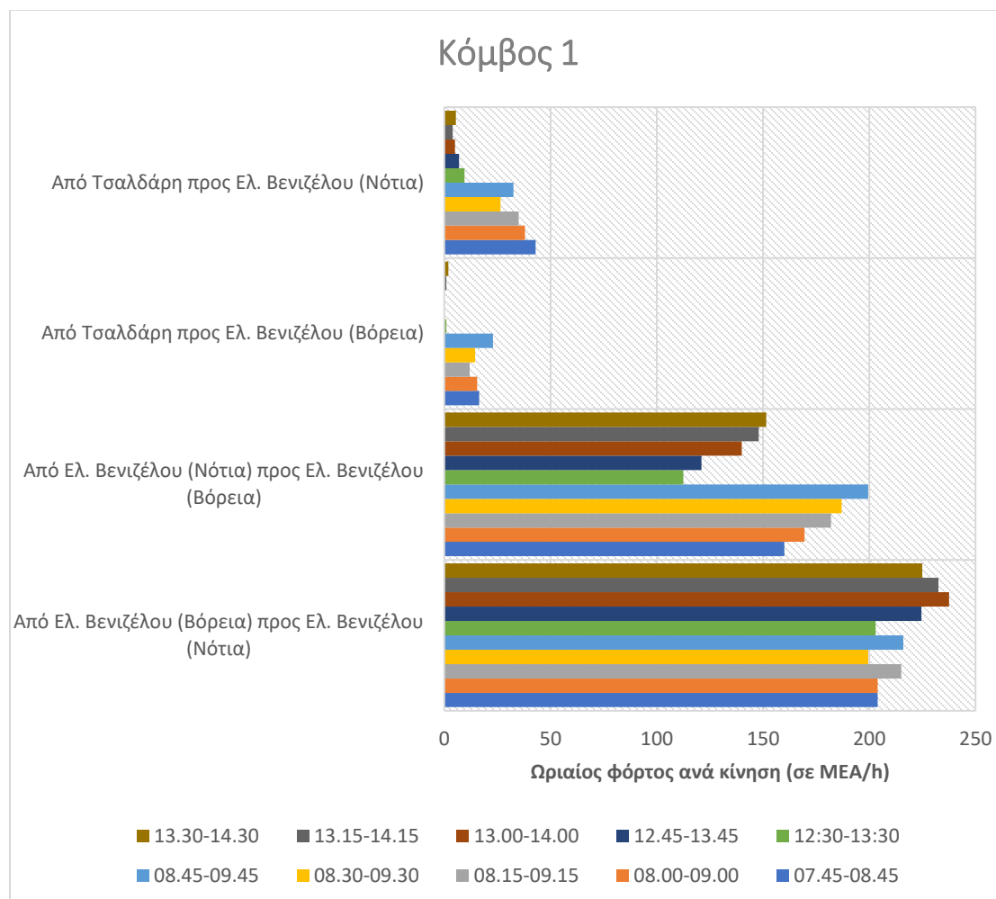
Διάγραμμα 5: Οπτικοποίηση αποτελεσμάτων κυκλοφοριακών ροών (ΜΕΑ/h) στον κόμβο 1
